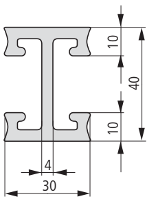
ダブルブスバー U-BAR-500/T
