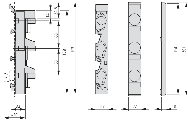
① 前面プレートサポート
