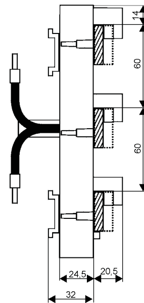
ダブルアダプタ Z-SS-60-ADD/6...
