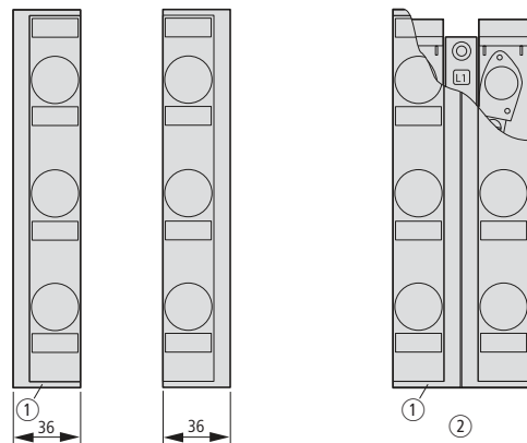
① 前面プレートサポート ② ブスバーサポートへの装着時
