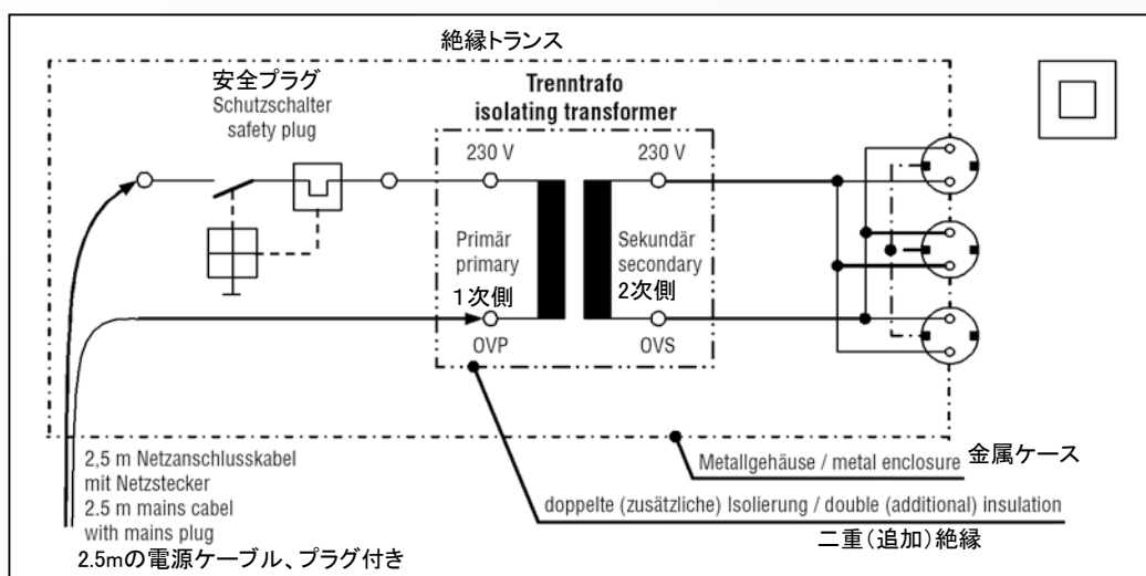
概略図
